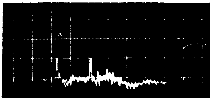
#294 C_7H_{16}/O_2 2P-100 P @ 5 cm (Vert.: 0.1 psi/div, Horiz.: 50 \mu sec/div)
