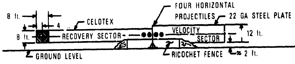
SECTION A-A
