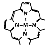
Metalloporphyrin
