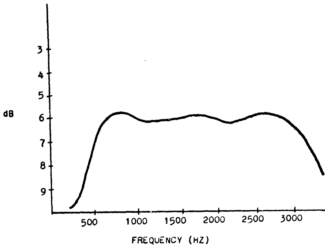
A. Actual Frequency Response
