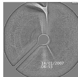
Video 4. doi:10.1016/j.icarus.2018.09.013.
