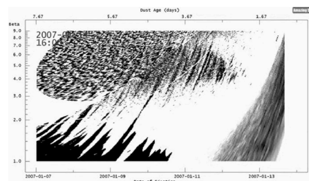
Video 6. doi:10.1016/j.icarus.2018.09.013.
