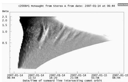
Video 8. doi:10.1016/j.icarus.2018.09.013 .
