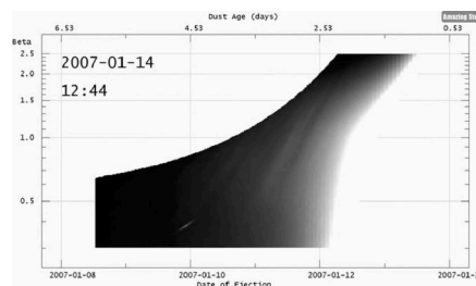
Video 10. doi:10.1016/j.icarus.2018.09.013 .
