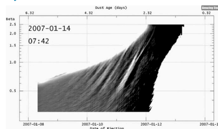
Video 1. doi:10.1016/j.icarus.2018.09.013.
