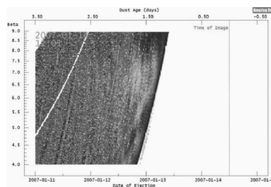
Video 7. doi:10.1016/j.icarus.2018.09.013.
