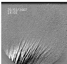
Video 3. doi:10.1016/j.icarus.2018.09.013.
