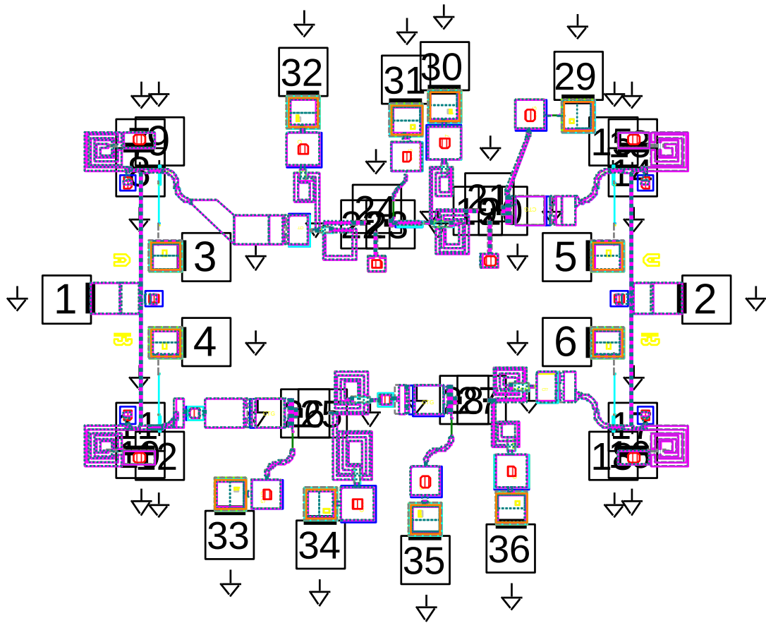
Fig. 48 2-D Axiem EM plot of T/R Module 2 (36 ports)
