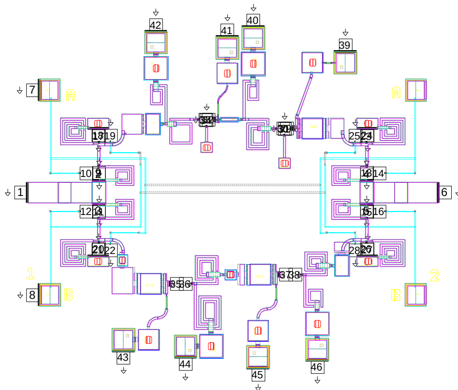
Fig. 41 2-D Axiem EM plot of T/R Module 3 (46 ports)
