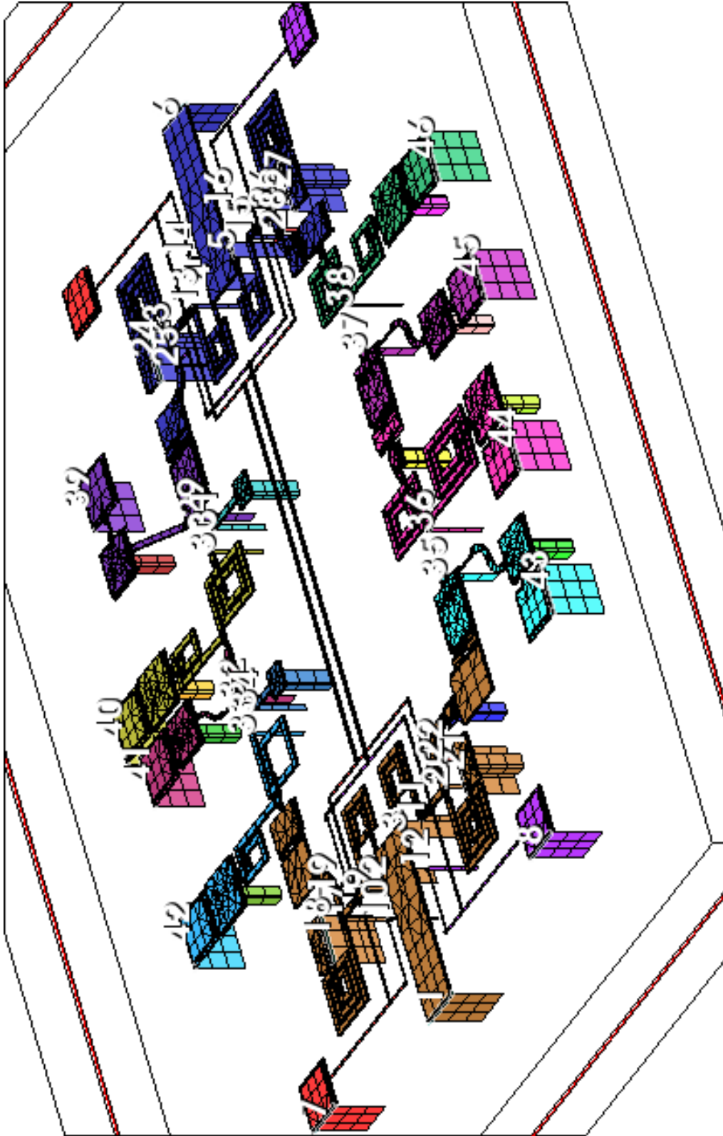
Fig. 42 3-D Axiem EM mesh plot of T/R Module 3 (46 ports)
