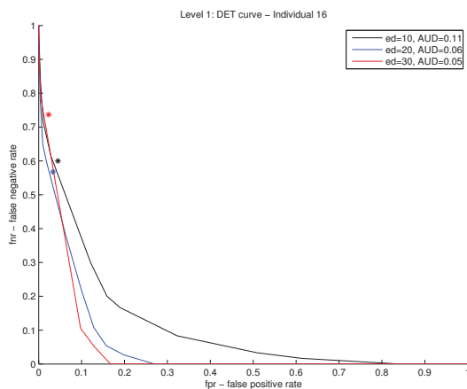
Fig. 4: DET curve.
