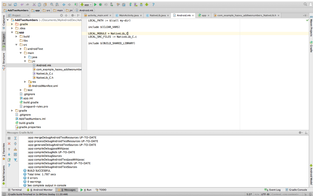
Fig. 12 Android.mk makefile
