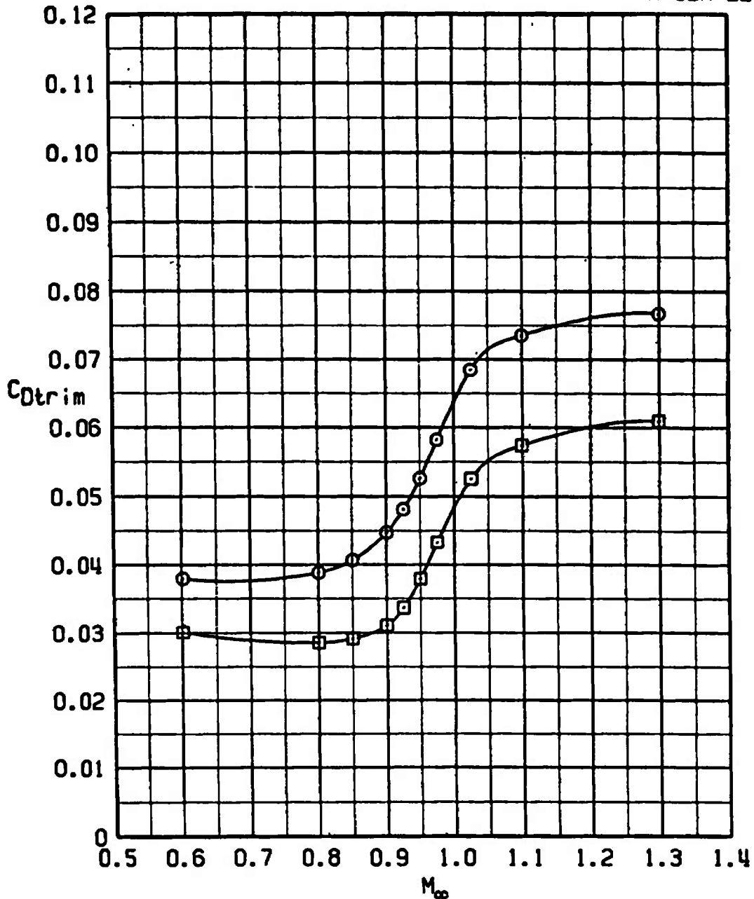
Figure 47. The effect of the SOM store on trim drag.
