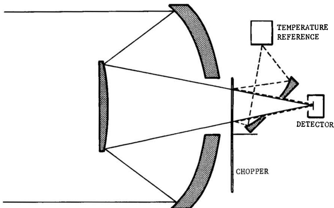
FIGURE 4-6. LWIR Radiometer
