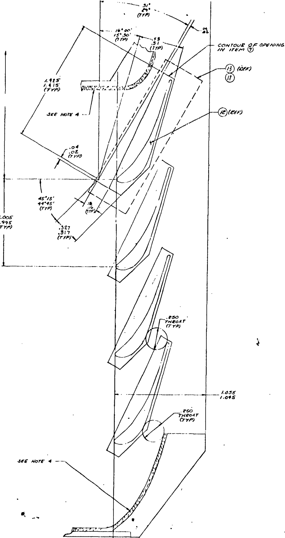
SECTION 13-13 SCALE: 5/1
