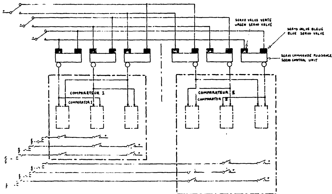
SURVEILLANCE DE LA COMMANDE D'ELEVONS INITIALE ELEVONS MONITORING SYSTEM (INITIAL DESIGN)
