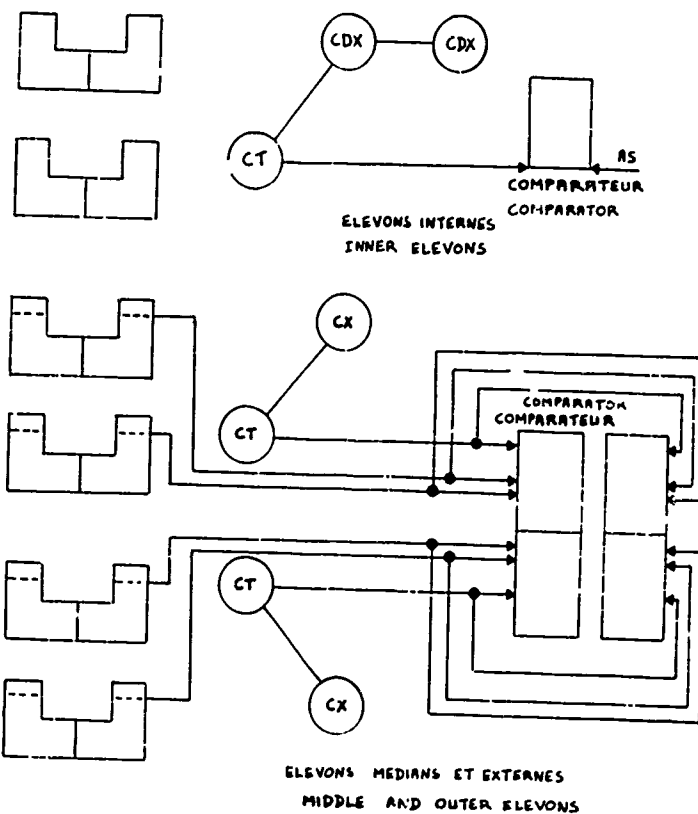
SURVEILLANCE DE LA COMMANDE D'ELEVONS MODIFIEE ELEVONS MONITORING SYSTEM (MODIFIED SOLUTION)
