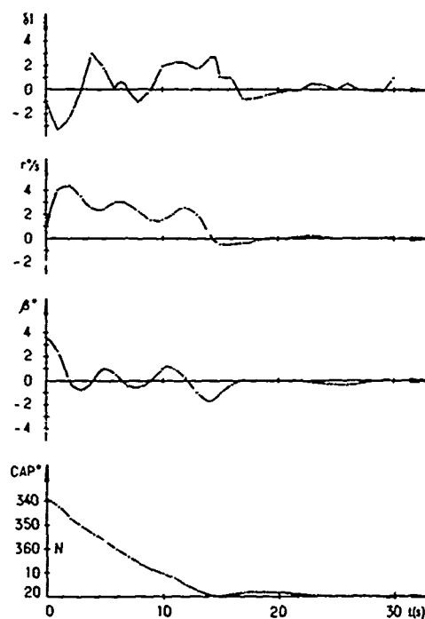
Avion avec bidons - Dérive agrandie Aircraft with tip tanks - Greater fin
