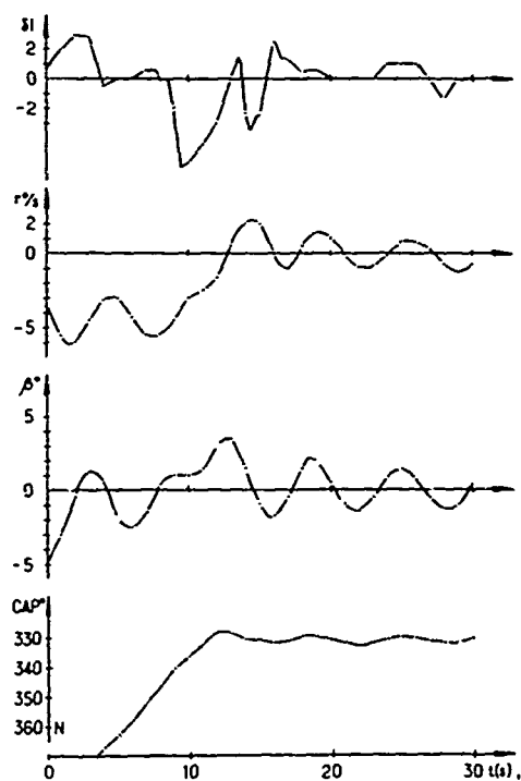
Avion avec bidons - Dérive initiale Aircraft with tip tanks - Normal fin
