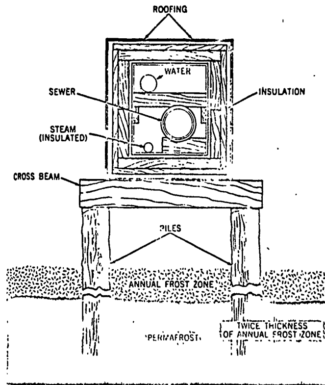
Figure 10. Utilidor. 7
