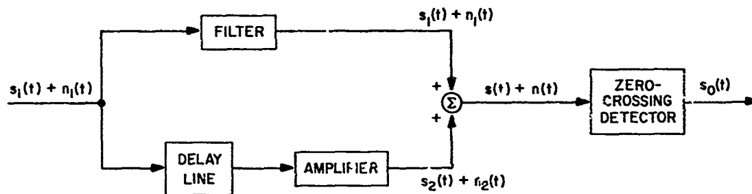
Fig. 4—Peak-amplitude estimator
