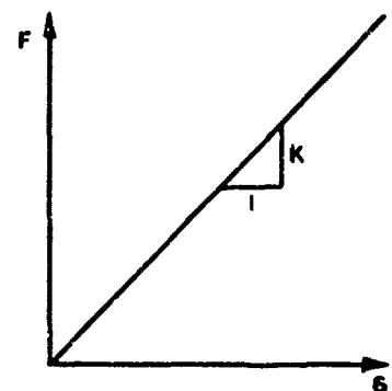
a. FORCE-DEFLECTION
