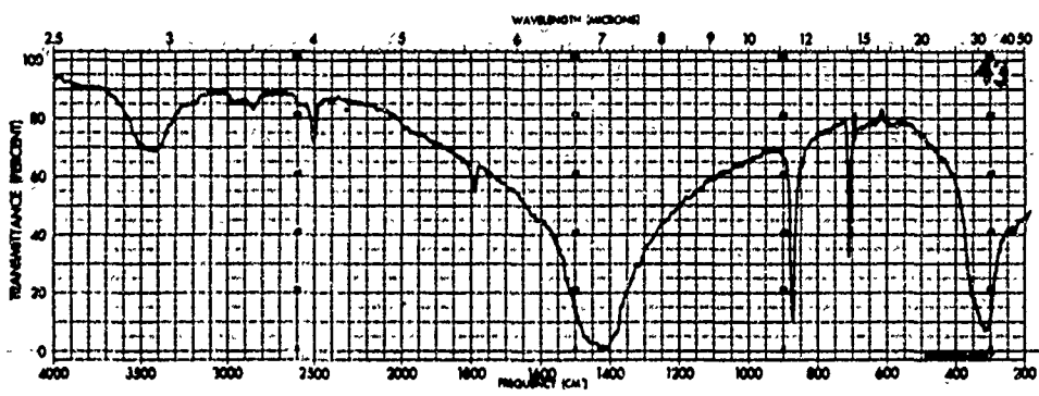
Misc. 4 Calcium carbonate CaCO 3
