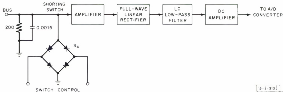
Fig. 4. Rectifier system.
