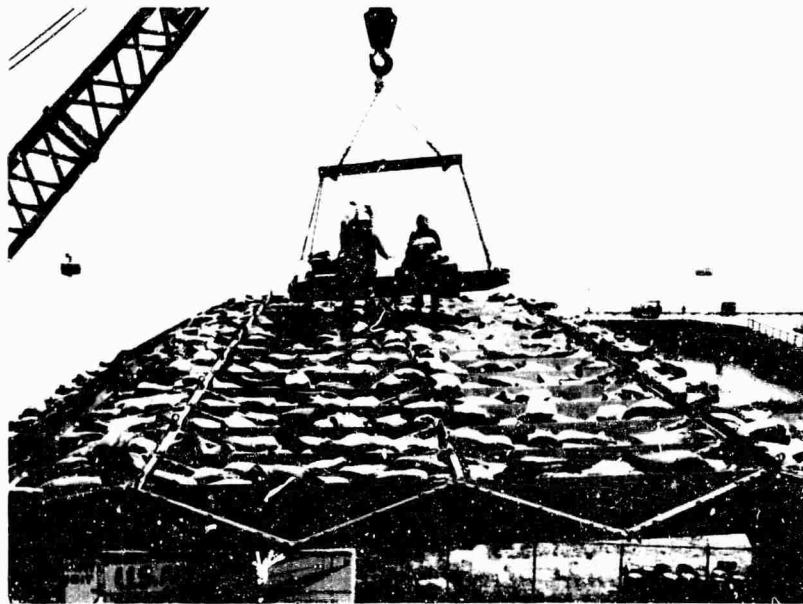
Fig. 53. Sandbag placement.
