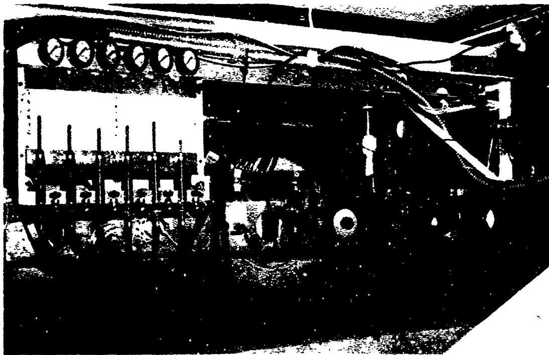
Fig. 17. Test setup
