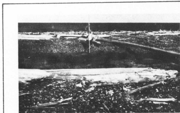
Fig. 35. Gravel Beach, (D9-17).
