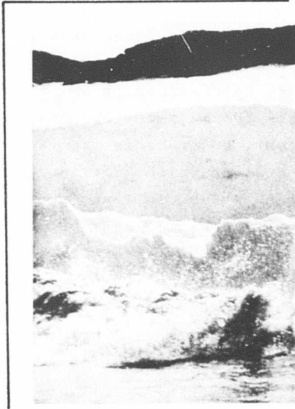
Fig. 15. Snowblock Collapse.
