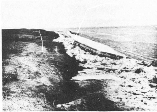
Fig. 56. Ice Shove (Colville).
