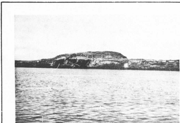
Fig. 46. Pingo (C1-32).
