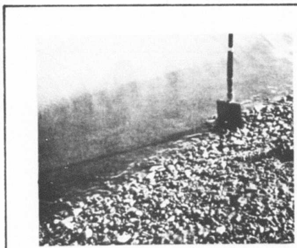
Fig. 35. Gravel Beach, (D9-17).
