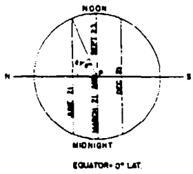
Figure 7. Position of the sun, latitude 0° latitude.
