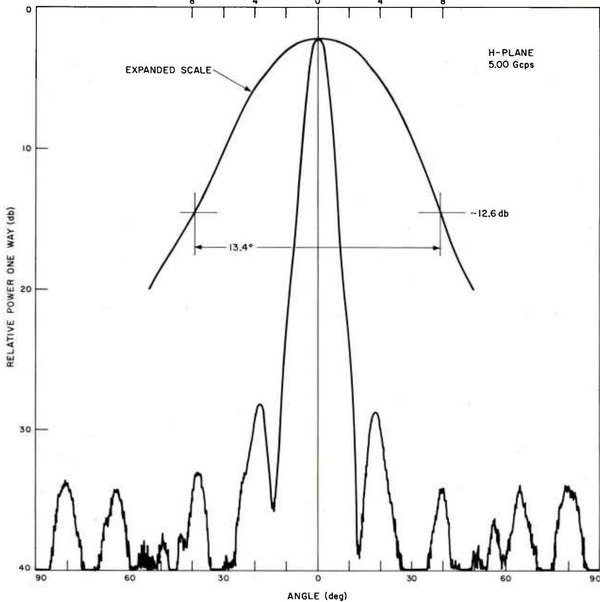
Fig. 7. Antenna pattern 5.0 Gcps H-plane.
