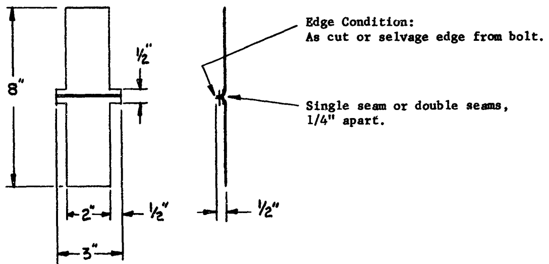
Fin Seams
