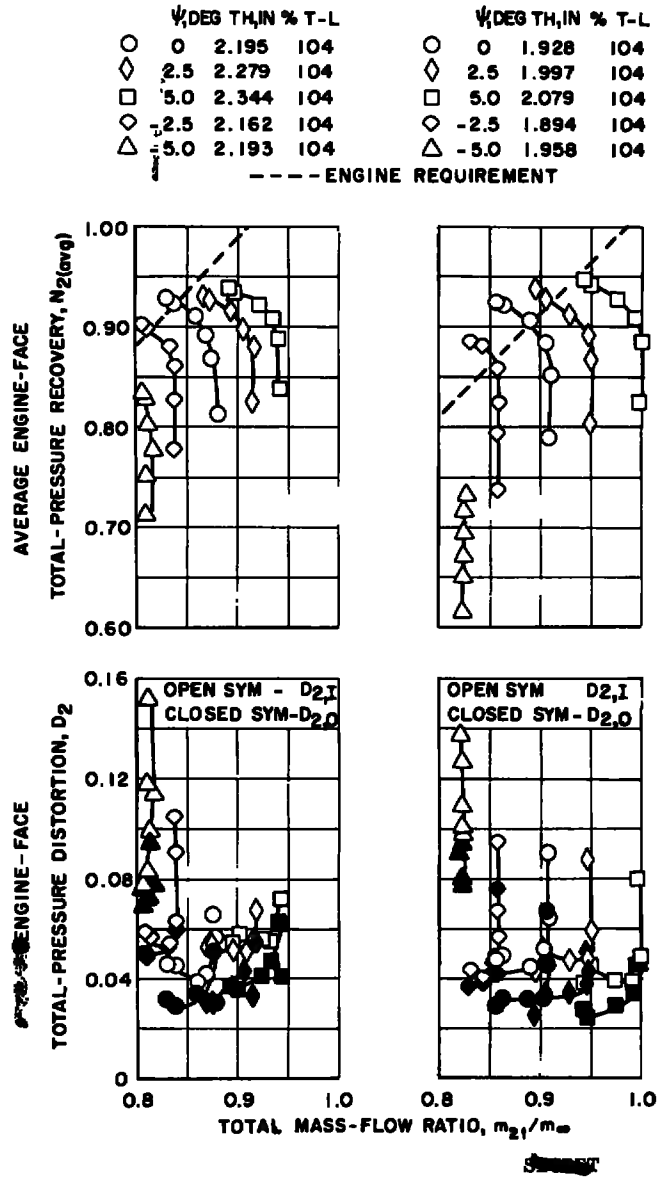
d. M_{\infty} = 2.00 , Configuration 19
